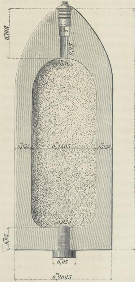
Fig. 4. — Obus du mortier rayé ou canon court. Coupe verticale suivant l'axe. (Réduction au qu.)
